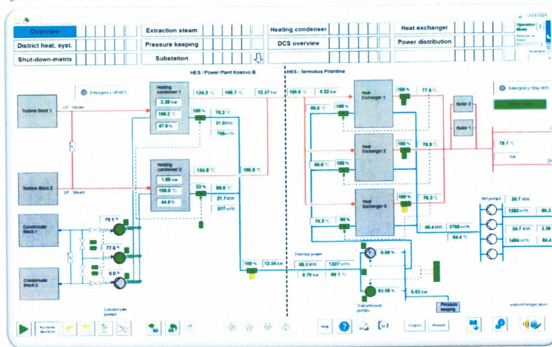
Figura 2. Skema e funksionimit të sisitemit të koogjenerimit
