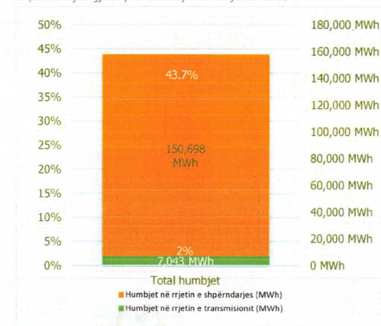
Figura 7. Humbjet në rrjetin e transmisionit dhe në rrjetin e shpërndarjes gjatë periudhës janar-dhjetor 2025
