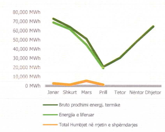
Figura 6. Energjia e prodhuar, e liferuar dhe humbjet MWh në janar-dhjetor 2025
