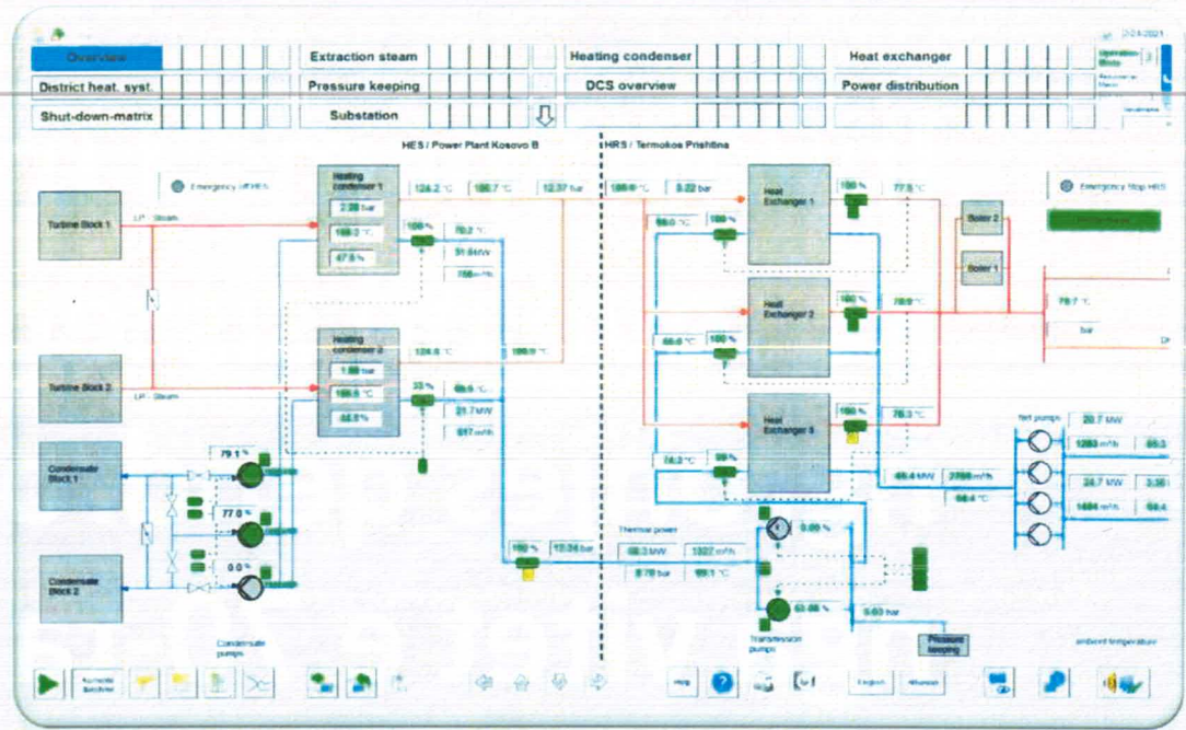
Figura 2. Skema e funksionimit të sistemit të koogjenerimit
