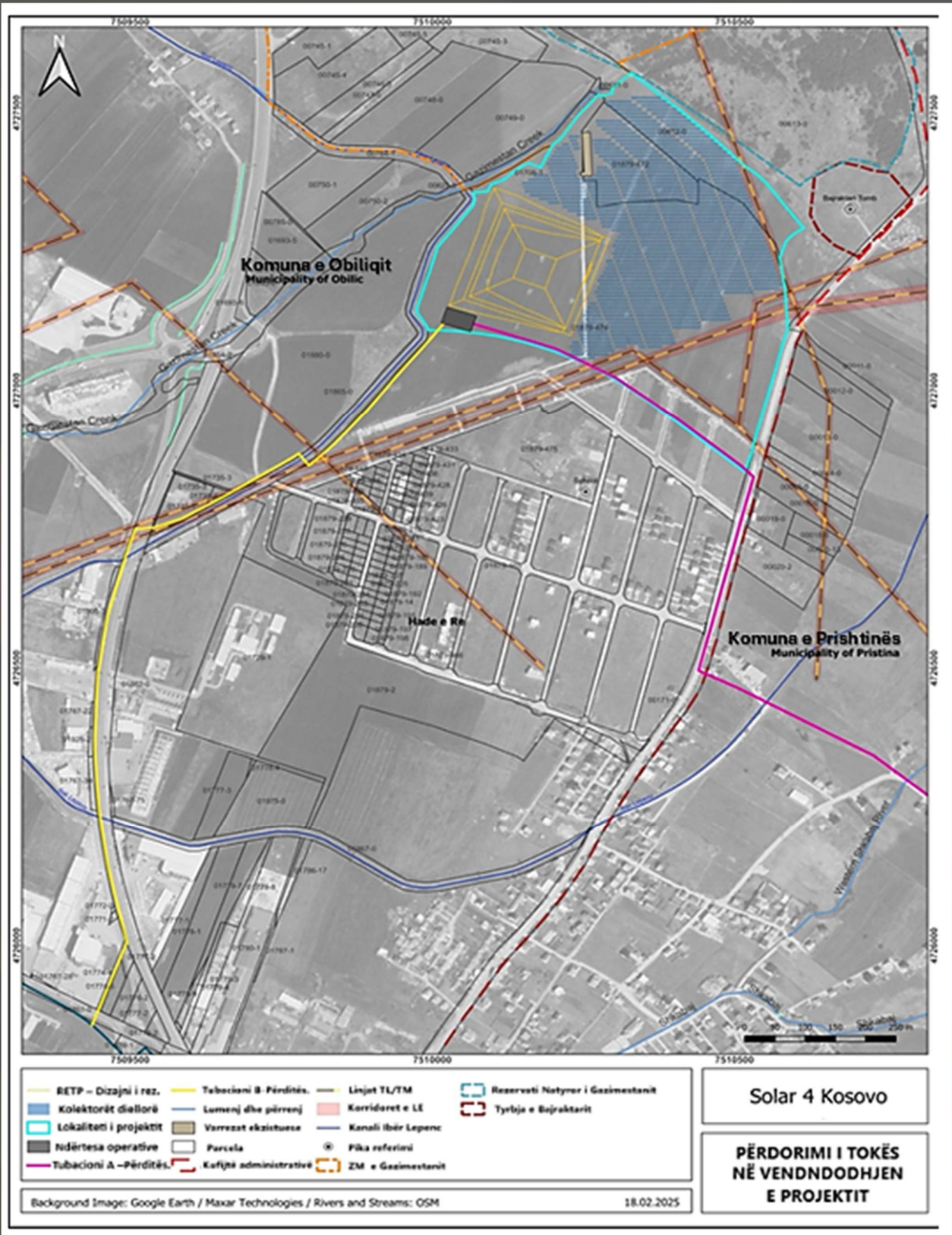
Harta e vendndodhjes së centralit termik diellor për projektin Solar4Kosovo II, e cila është subjekt i ndryshimeve në dizajn për Pipedinën B, pasi rruga ende nuk është finalizuar.
