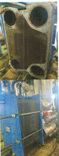
Figura 3. Dëmontimi/montimi i këmbësyt të nxehësissë 4 pas pastimit kimik në termonënstacionin e Bregu I Diellit.
