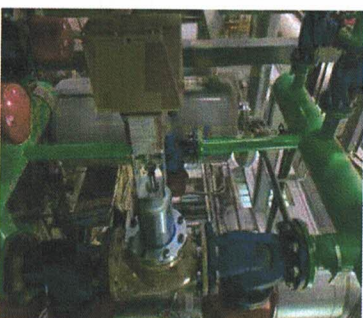
Figura 8. Ndërimi i valvës DN 125 e cila ishte në defekt, Check valve të paisja për mbajtje të presionit në rrjet të kogjenierimit.
