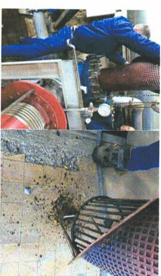
Figura 6. Pastrimi i filterave: NQ, HES, dhe stacion BD.
